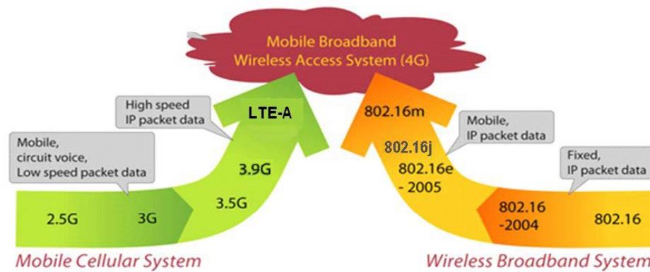
圖 5：IMT-Advanced 技術趨勢衍進
